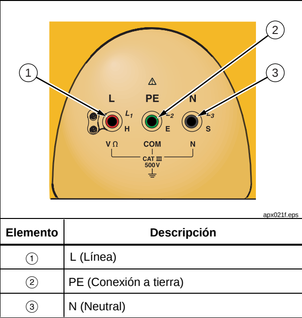
Figure 4. Terminales de entrada
