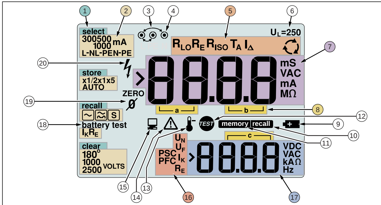
Figura 3. Características de la pantalla
