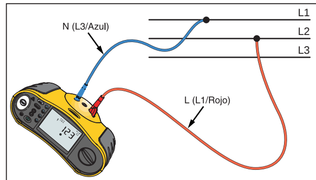
Figura 14. Medición en un sistema trifásico
