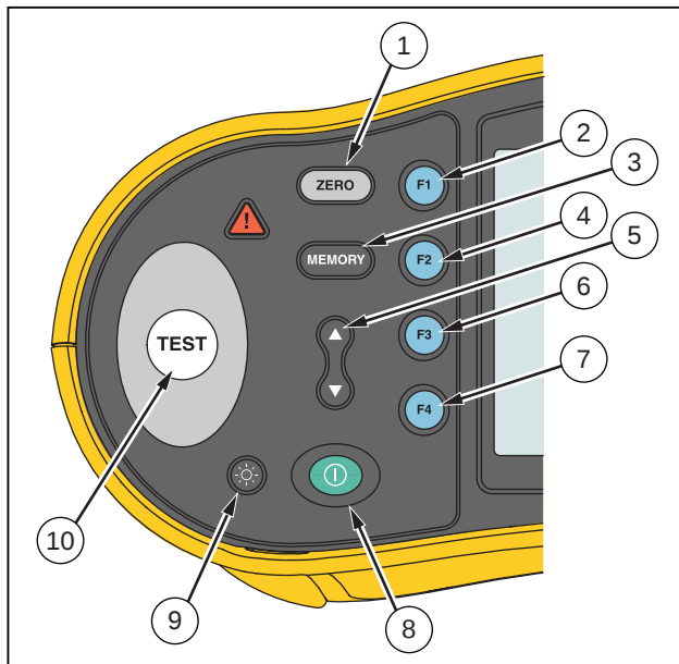
Figura 2. Botones pulsadores
