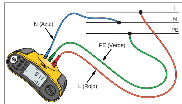
Figura 12. Conexión trifilar para prueba de lazo de resistencia de tierra
