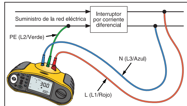
Figura 17. Conexión para comprobaciones de interruptores por corriente diferencial en sistemas eléctricos de TI
