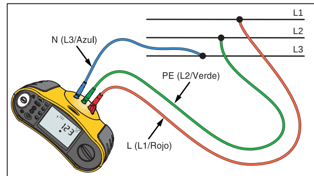
Figura 21. Conexión de prueba de secuencia de fases
