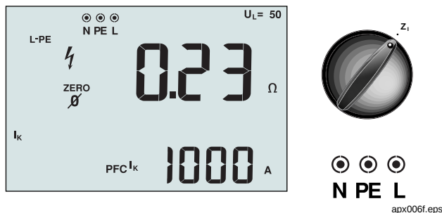
Figura 10. Impedancia de lazo/línea/Configuración de interruptor y terminal
